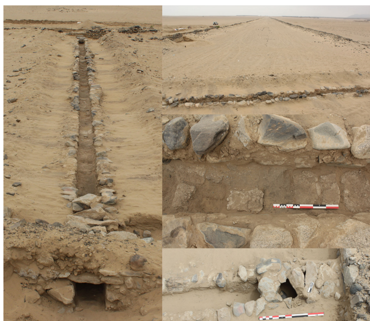
Figura 6. Detalle de las excavaciones realizadas en el CMP-1. Véase el canal que atraviesa el camino, su sistema de esclusas para pasar entre los muros, así como la base con greda en el fondo del canal y la cubierta de piedras para proteger el canal y el agua de los transeúntes.
