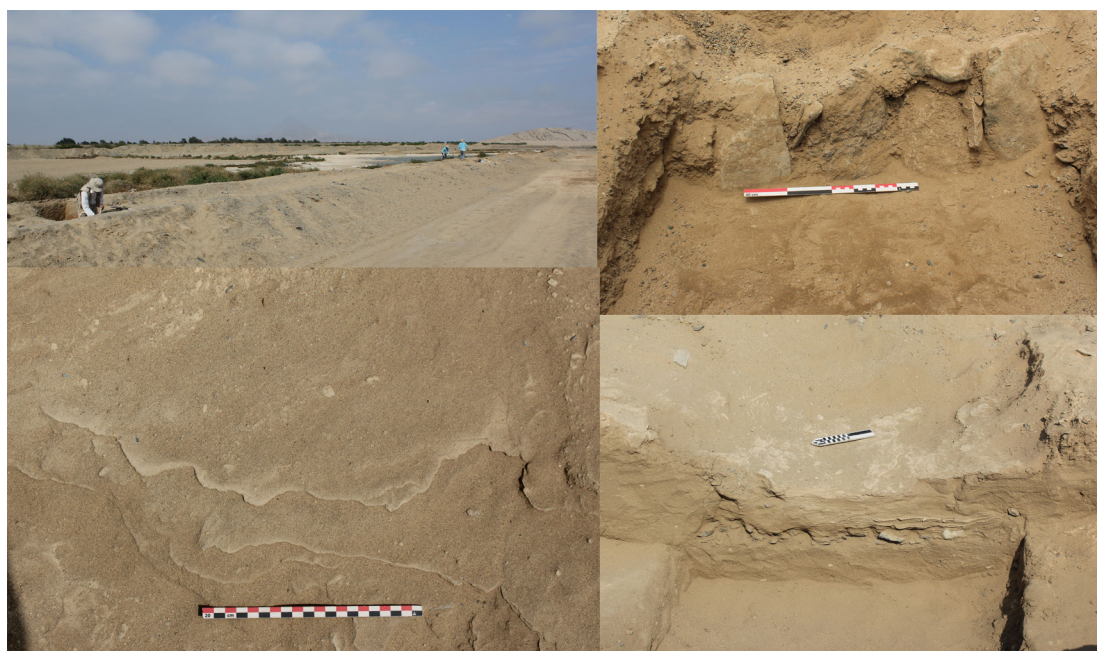
Figura 8. Detalle de las excavaciones del canal elevado del sector campos de cultivo Chimú al NW de Cerro La Virgen en Huanchaco. Véase el muro de piedras solo presente en la cara oeste del canal y los sedimentos laminados que confirman la existencia de flujos de agua en el pasado.
